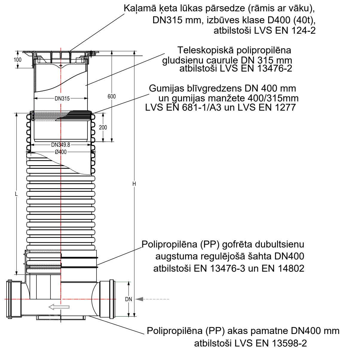
PP akas DN400 vāka izbūve zālāja segumā
