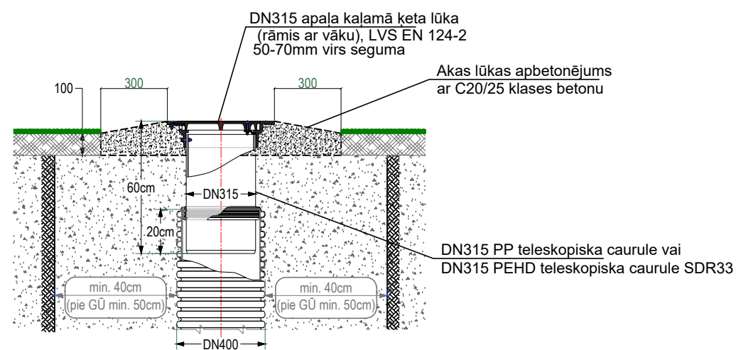
PP akas DN400 vāka izbūve zālāja segumā
