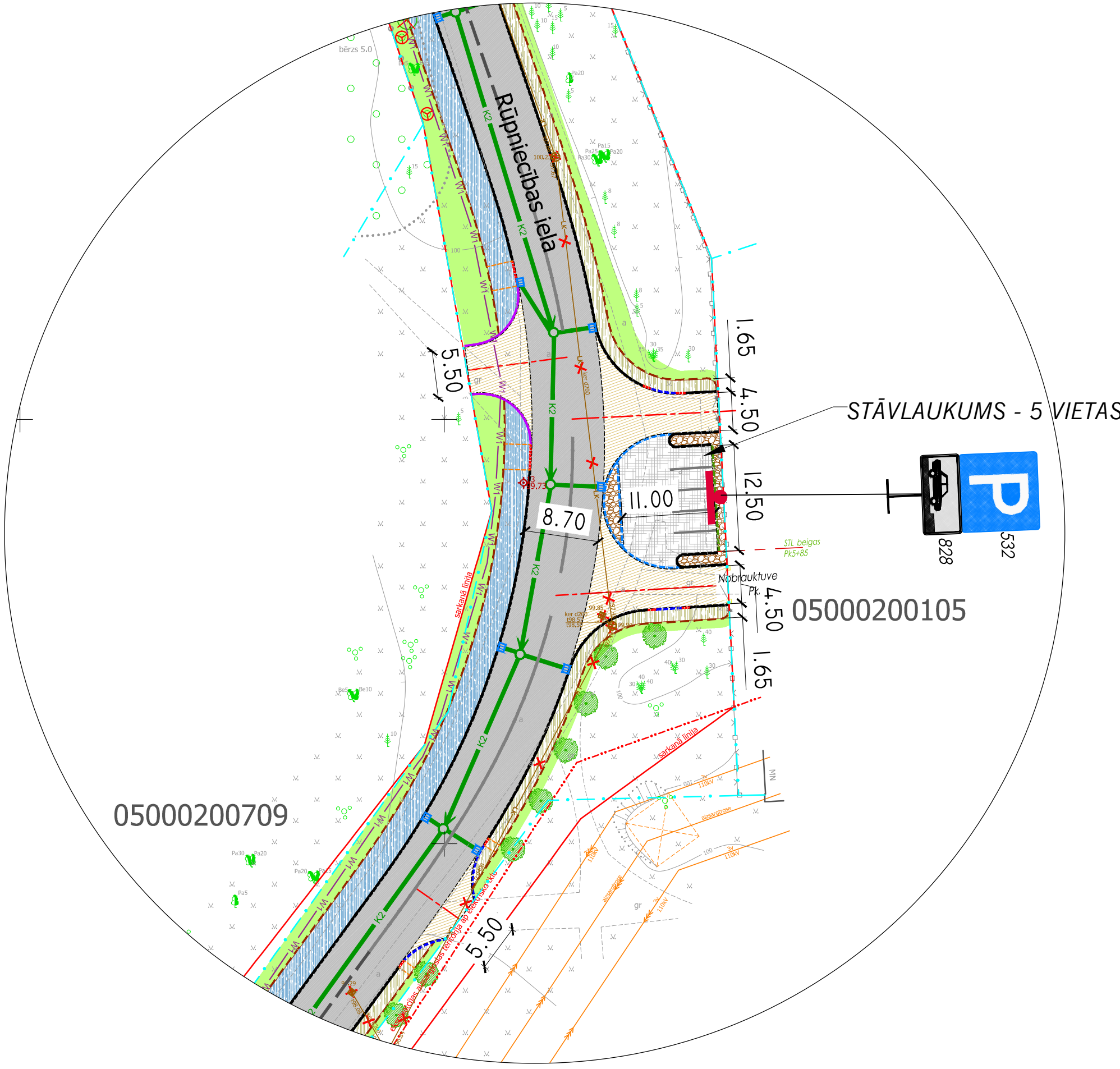
MEZGLS B M1:500
