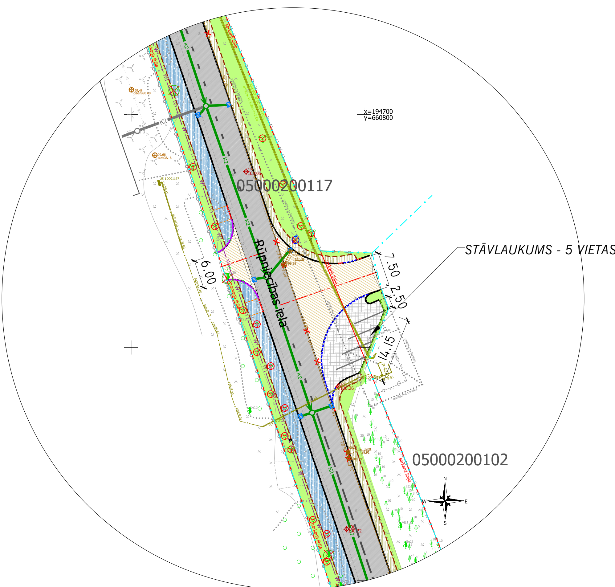
MEZGLS A M1:500
